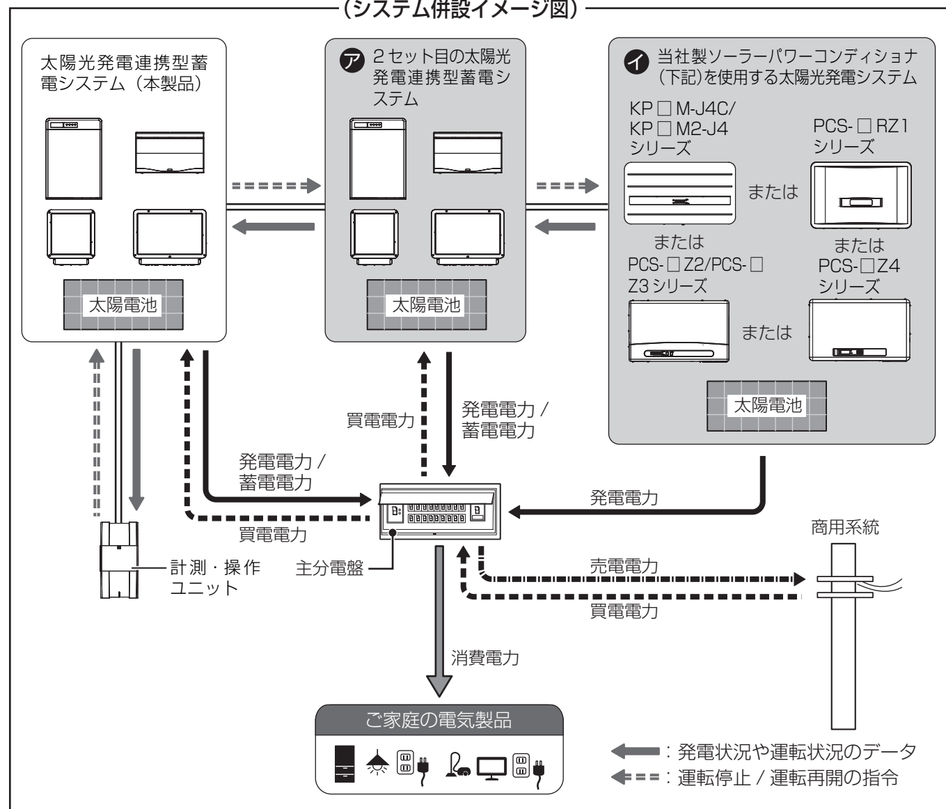
（システム併設イメージ図）
